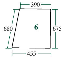
21/4041-5 (D7048/F) Lateral (Fija, ambos lados) Side (Fixed, LH or RH)
