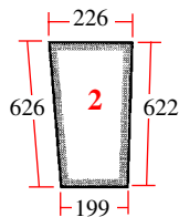
20/4015-2 (D7042, K965469) Avant (gauche) Front (LH)
