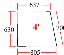
20/4039-6 (D7027, K303701) Porte (gauche) Door (LH)
