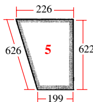
20/4037-1 (D7046, K965485) Porte (bas gauche) Door (LH lower)
