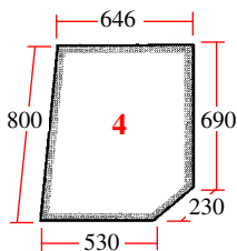
25/4035-1 (D.7044, 3125457R1) Porte (haut gauche) Door (LH upper)
