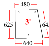
20/4043-2 (D7024, K303705) Côté (gauche) Side (LH)
