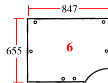
25/4072-33 (D.7099, 126317A1) Arrière (supérieur) avec découpe Rear (upper) with cut out
